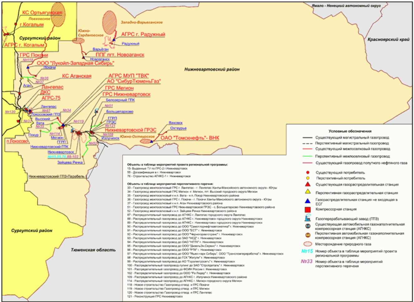
Схема расположения объектов газоснабжения Октябрьского муниципального района автономного округа
