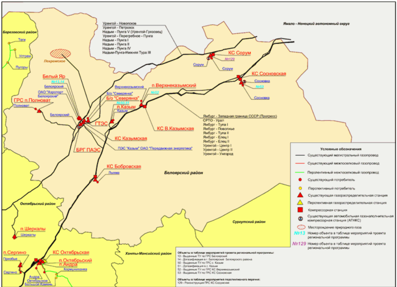
Схема расположения объектов газоснабжения Кондинского муниципального района автономного округа
