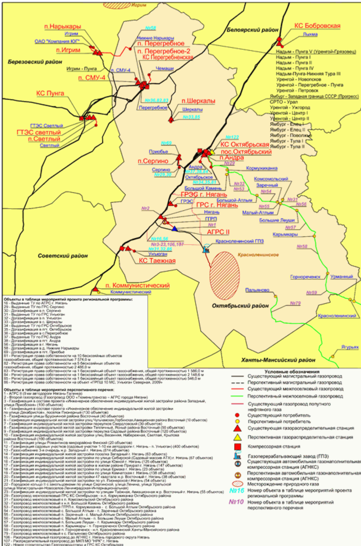
Схема расположения объектов газоснабжения Советского муниципального района автономного округа
