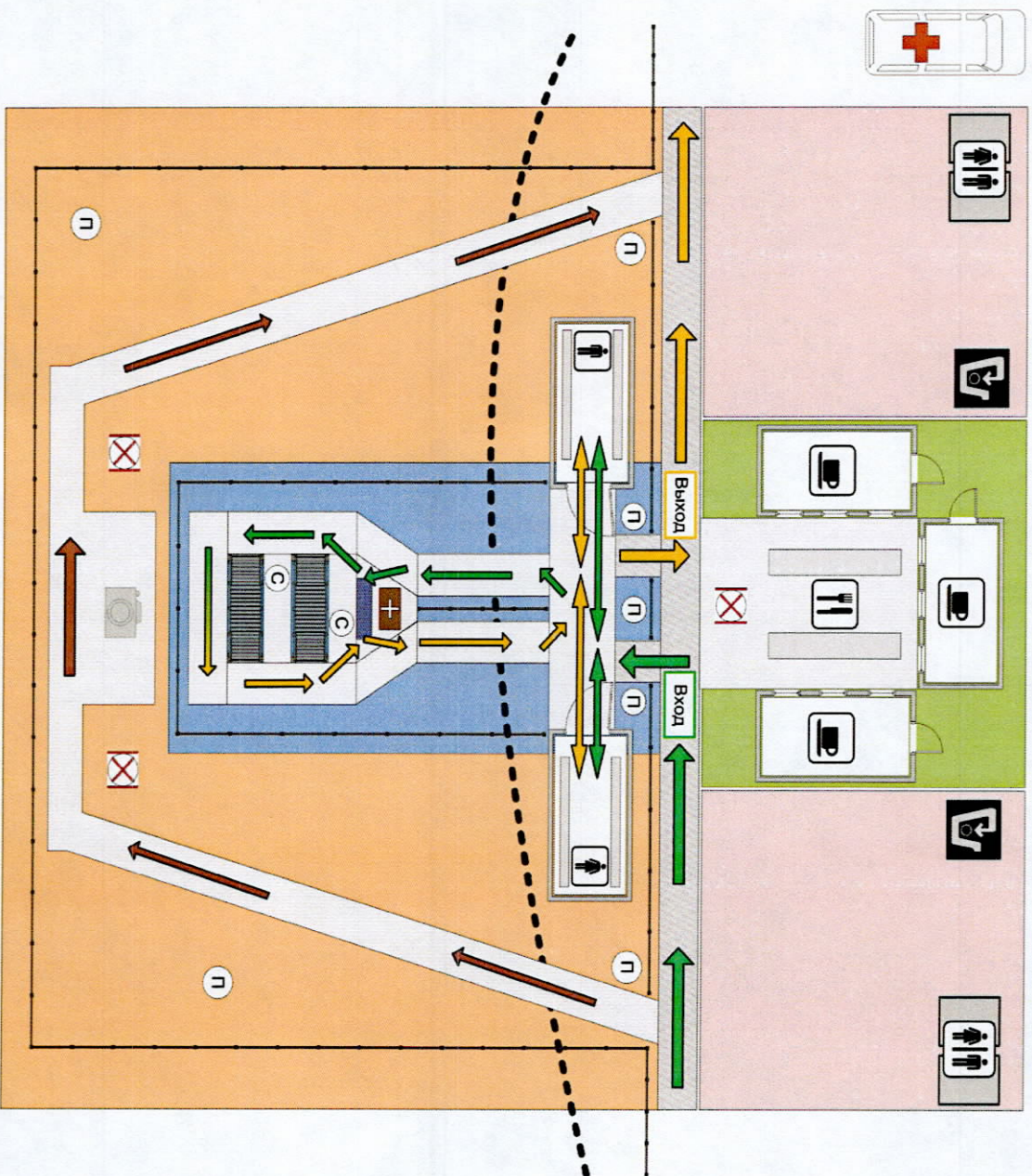
Схема организации Крещенских купаний с прорубью (майной) на 2 хода
