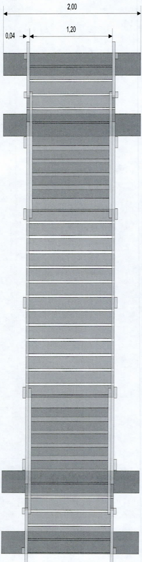
Чертеж конструкций мостков для Крещенских купаний на водных объектах (вариант 2)
