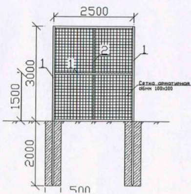
Торцевая секция
