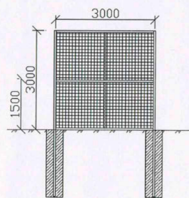
Рядовая секция
