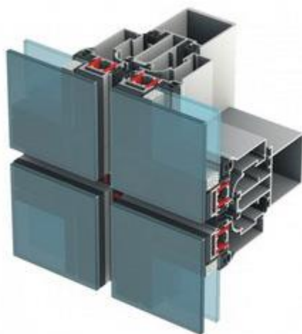
Рисунок 5.6 – Фрагмент структурного остекления
