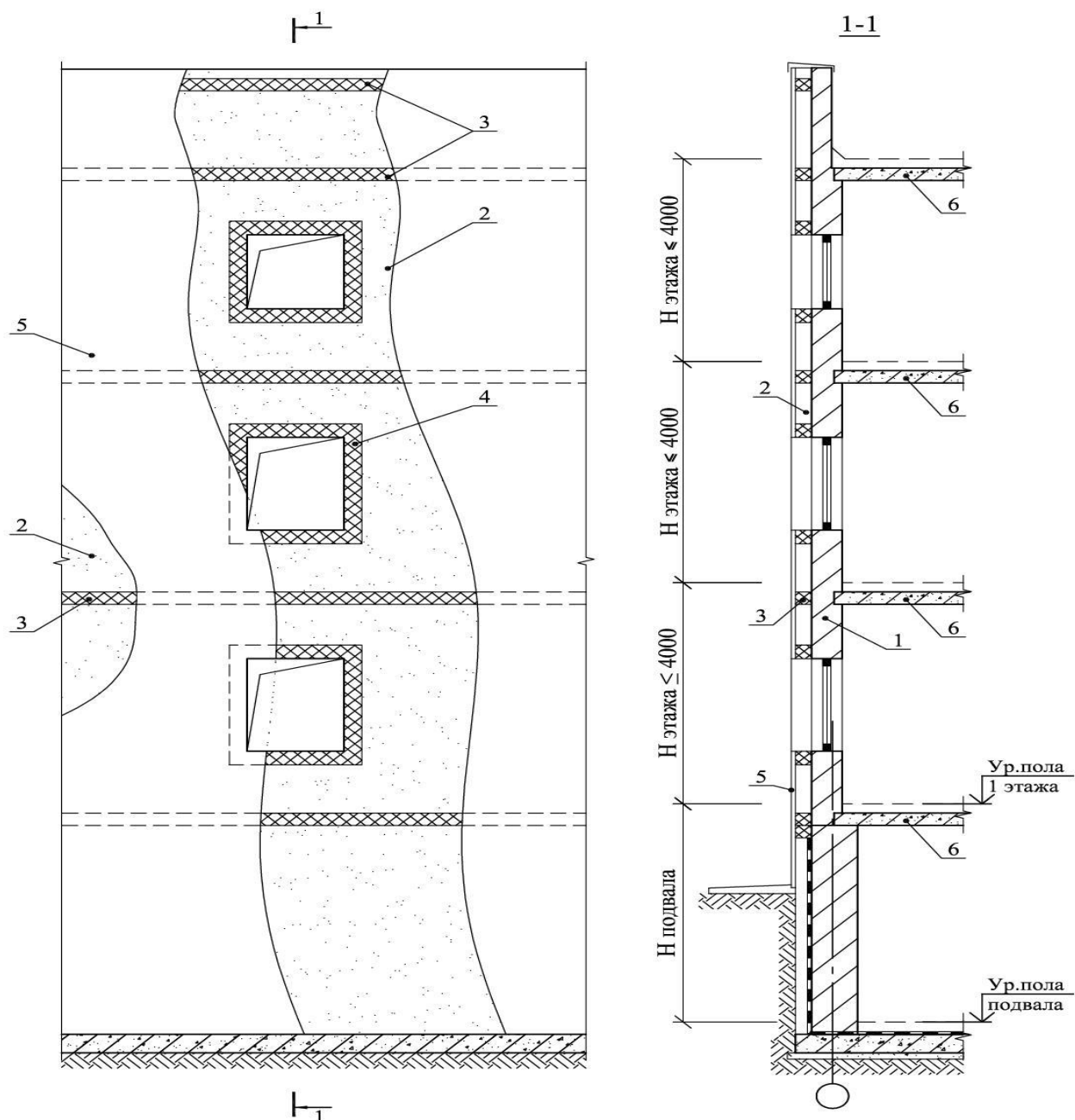
Рисунок 5.13 Устройство расщек в фасадной системе с защитно-декоративным слоем из тонкой штукатурки
