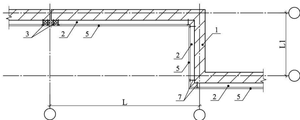
Рисунок 5.12 Устройство горизонтальных и вертикальных рассечек в фасадной системе.
