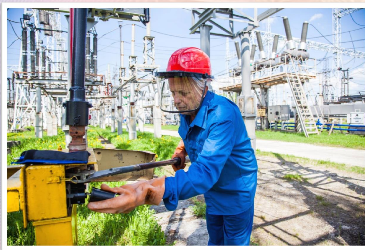
«Операция включения заземляющего ножа»
